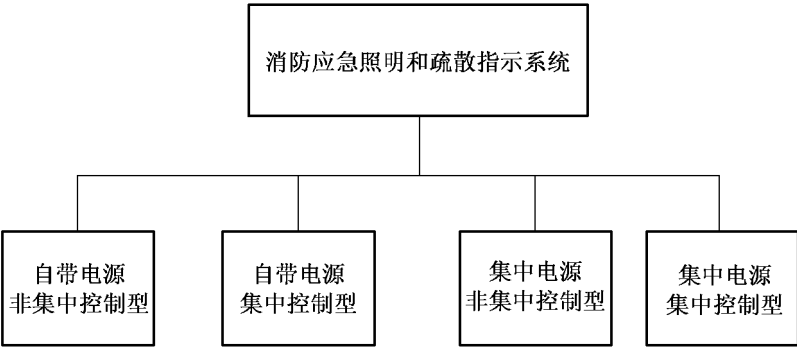
图 A.1 消防应急照明和疏散指示系统组成
