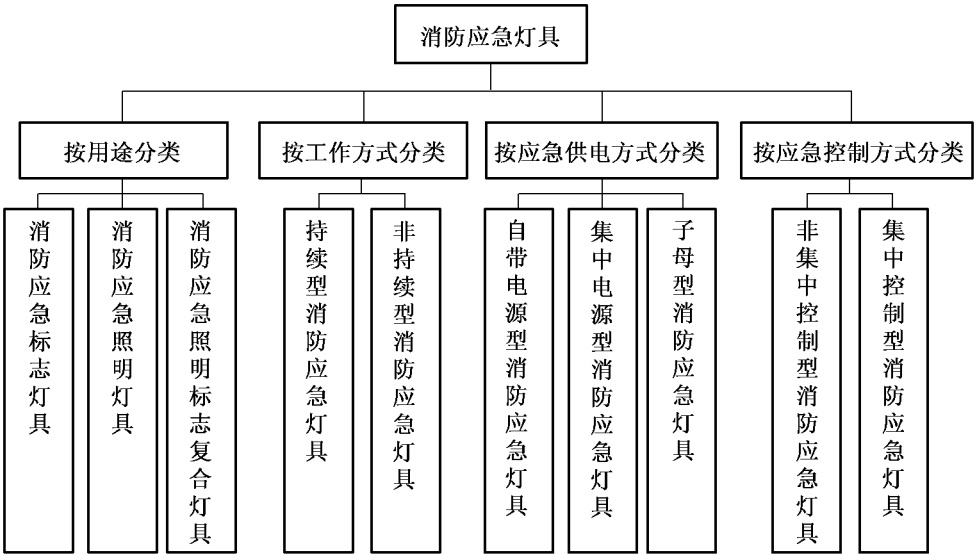
图 A.6 消防应急灯具组成
